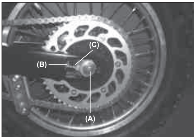
(A). Eje trasero. (B). Tuerca ajustadora. (C). Ajustador cadena.
