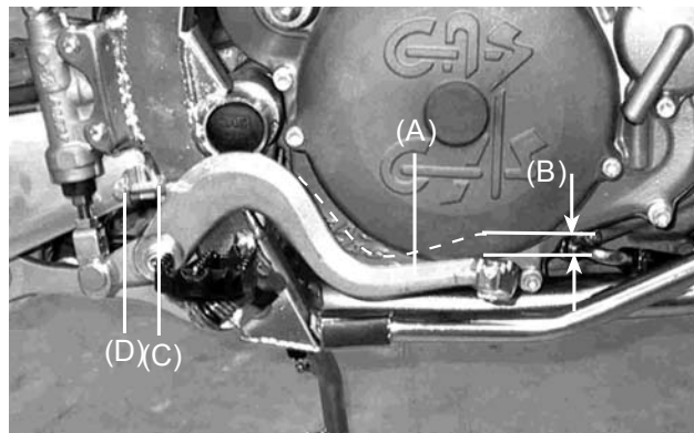
(A). Pedal freno. (B). 10 mm de juego. (C). Tornillo ajustador (D). Tuerca bloqueo.
