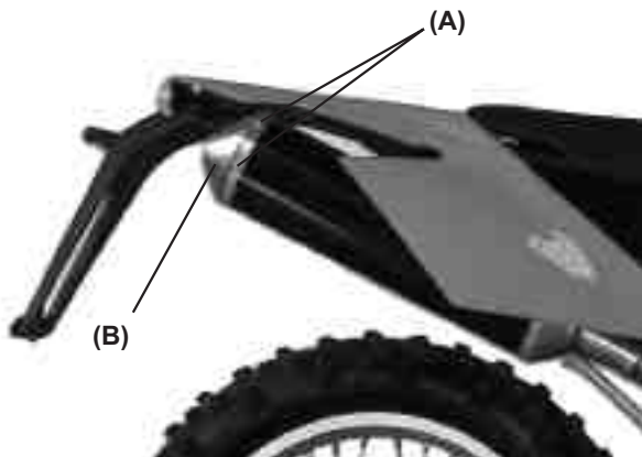
(A). Rivets. (B). Cache.
