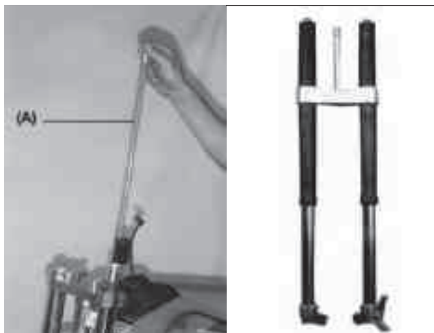
(A). Tige de l'hydraulique.
