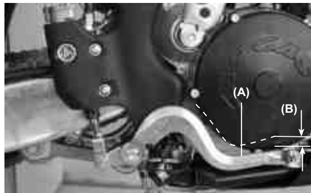
(A). Pédale de frein. (B). 10 mm de jeu.
