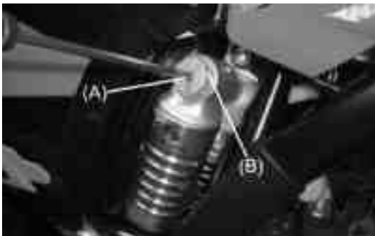
(A). Ajusteur de basse compression. (B). Ajusteur de haute compression.
