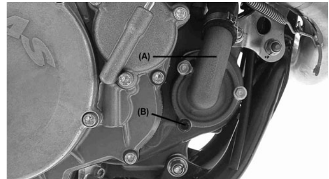
(A). Cache de la pompe à eau. (B). Bouchon de vidange du liquide de refroidissement.
