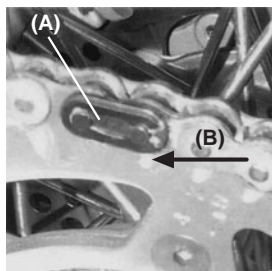
(A). Attache rapide. (B). Sens de rotation.
