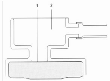
(1). Niveau du liquide. (2). Ouverture de remplissage
